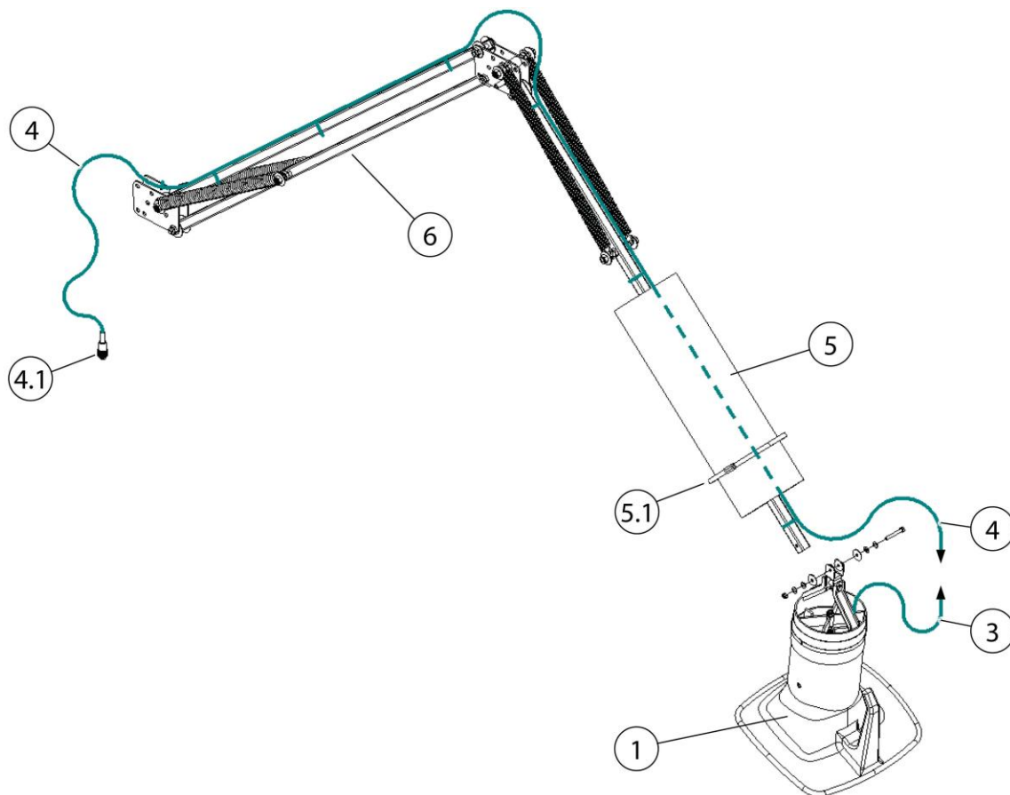
Abb. 19: Kabelverlegung - Absaugarm 2-4 Meter
