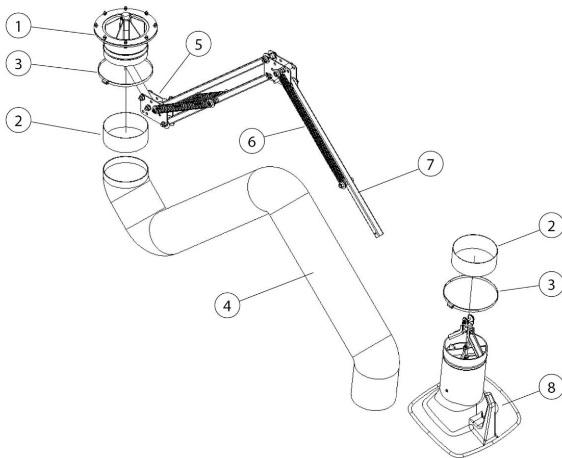
Abb. 3: Absaugarm
