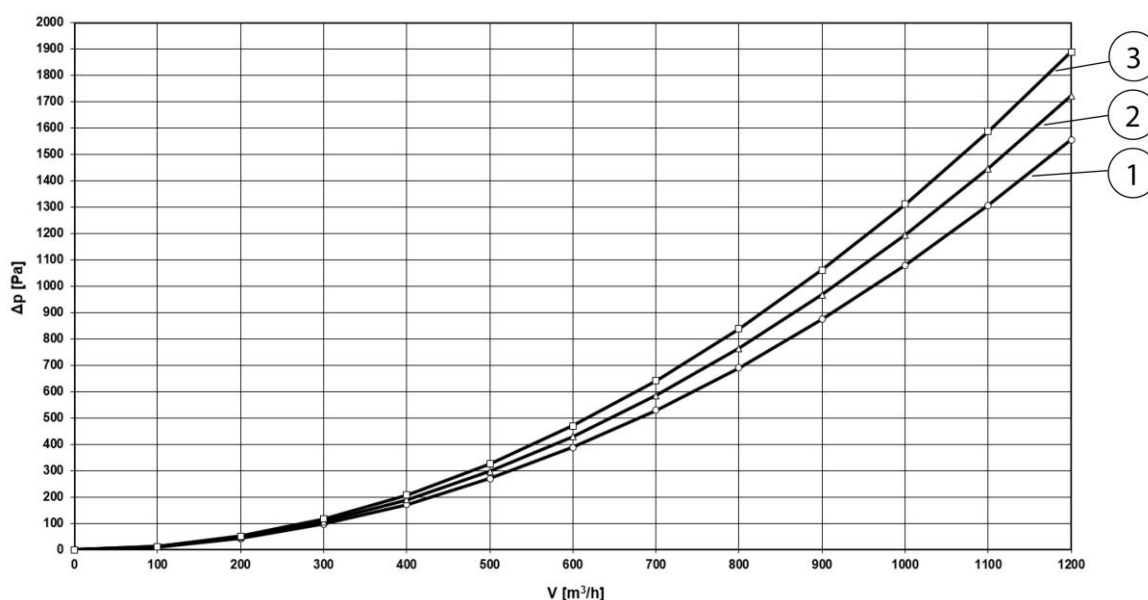
Abb. 21: Druckverlustdiagramm
