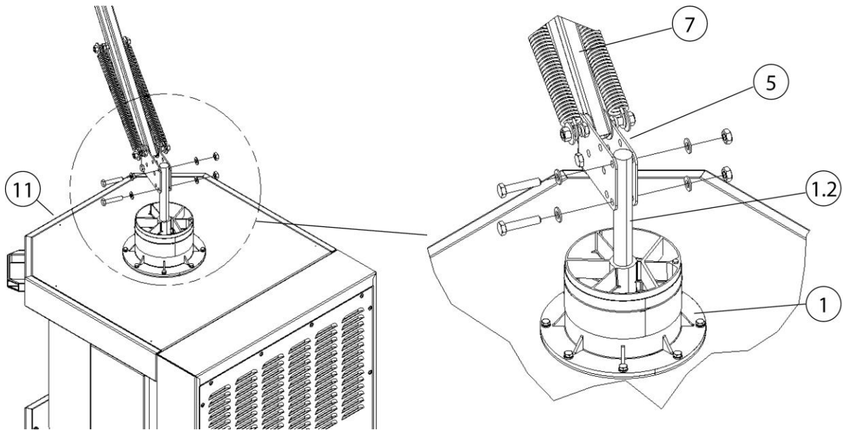
Abb. 9: Montage Tragegestell
