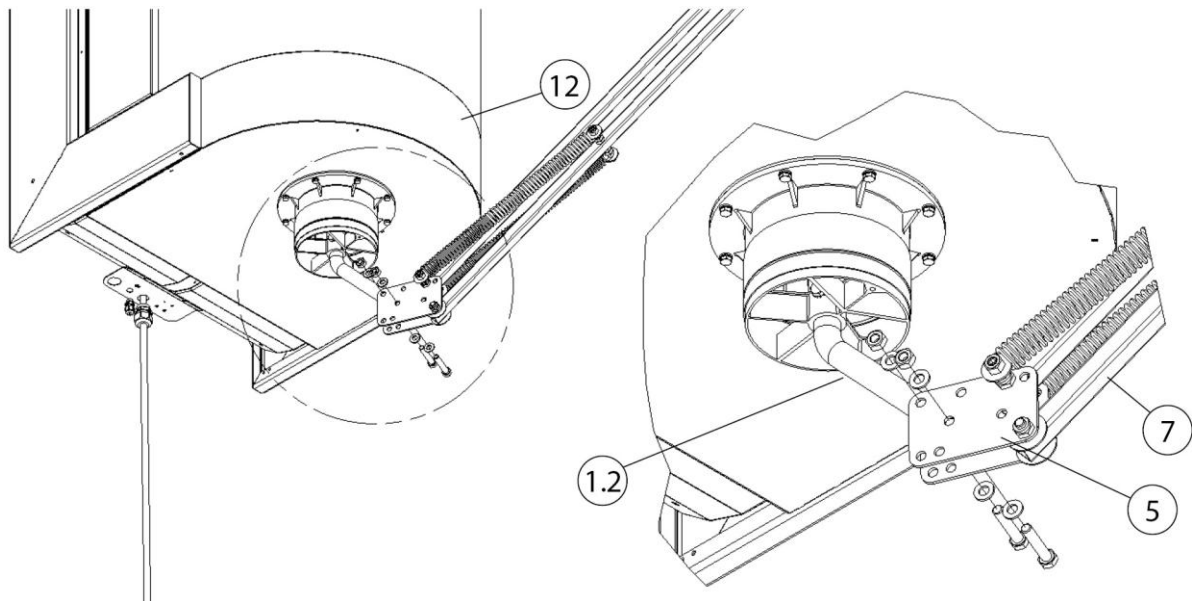
Abb. 11: Montage Tragegestell
