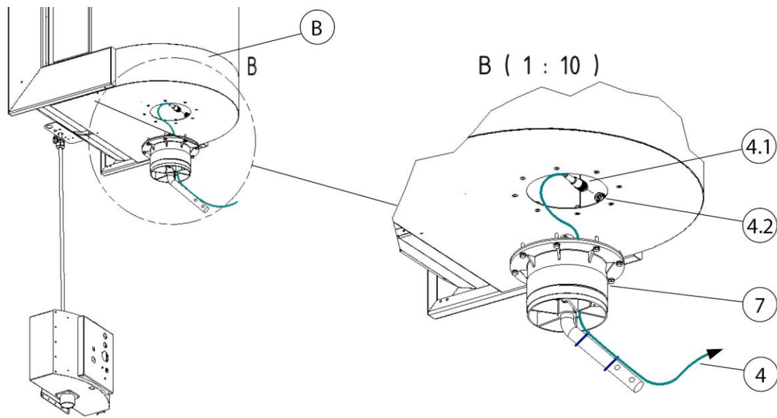
Abb. 17: Anschluss – stationäres Filtergerät
