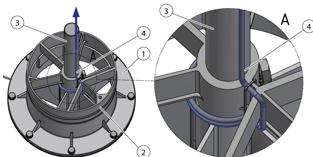
Abb. 15: Drehkranz
