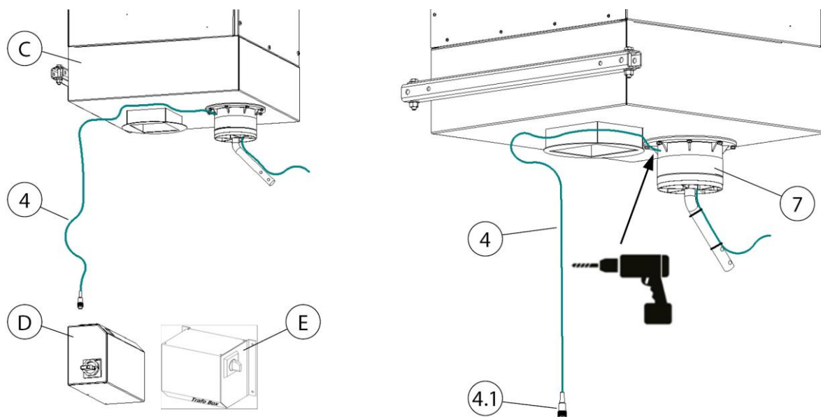
Abb. 18: Kabelverlegung – stationäres Gerät
