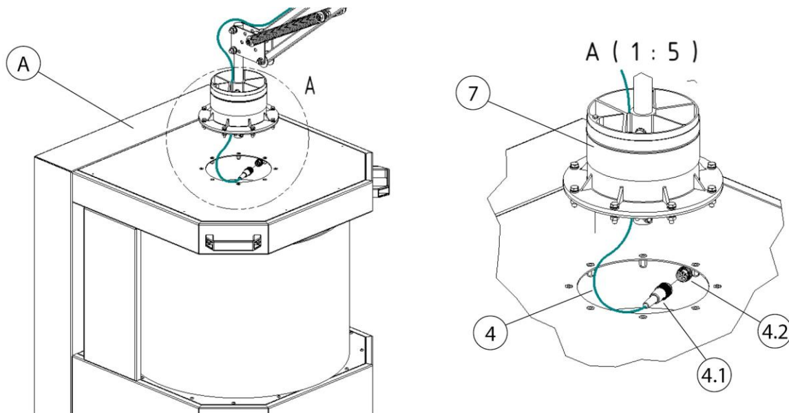
Abb. 16: Anschluss – mobiles Filtergerät
