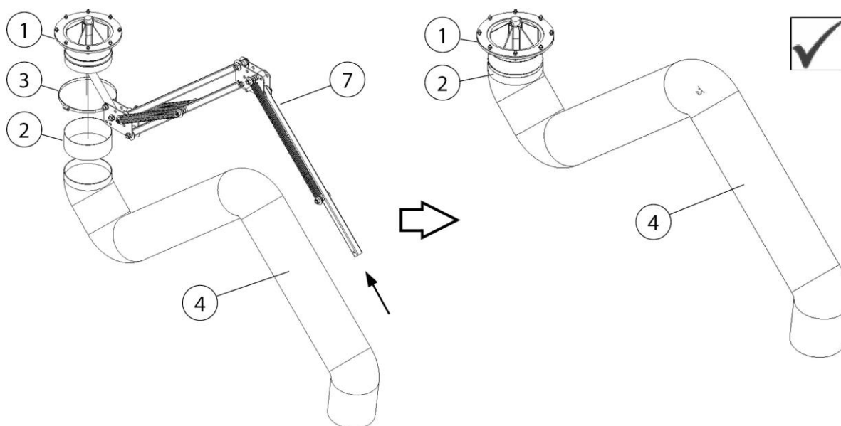
Abb. 13: Tragegestell/ Absaugarm
