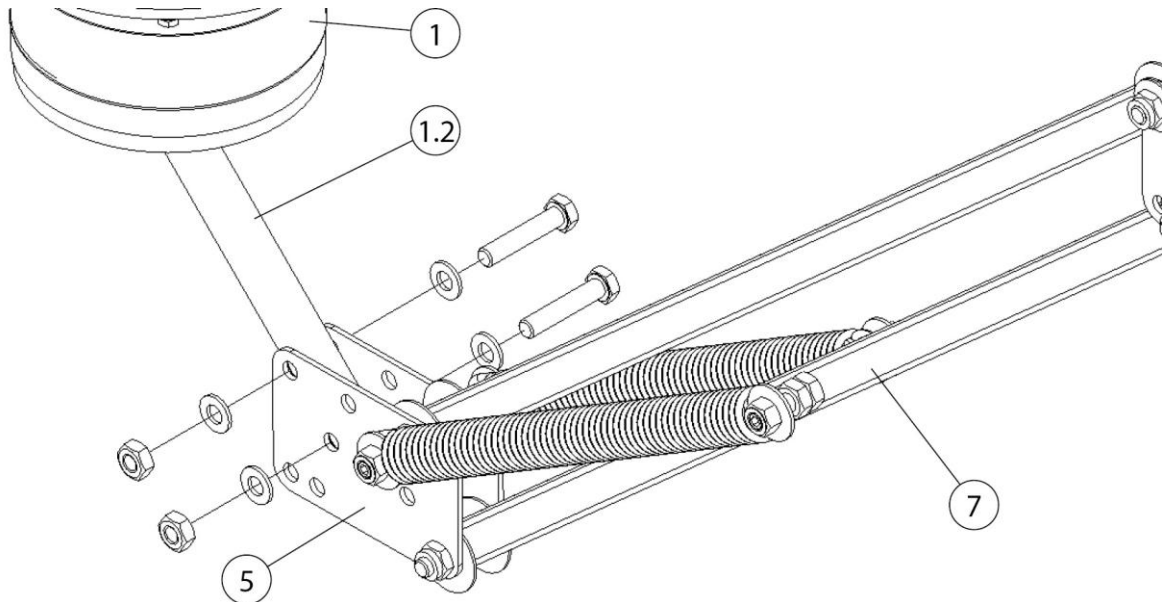
Abb. 6: Montage Tragegestell
