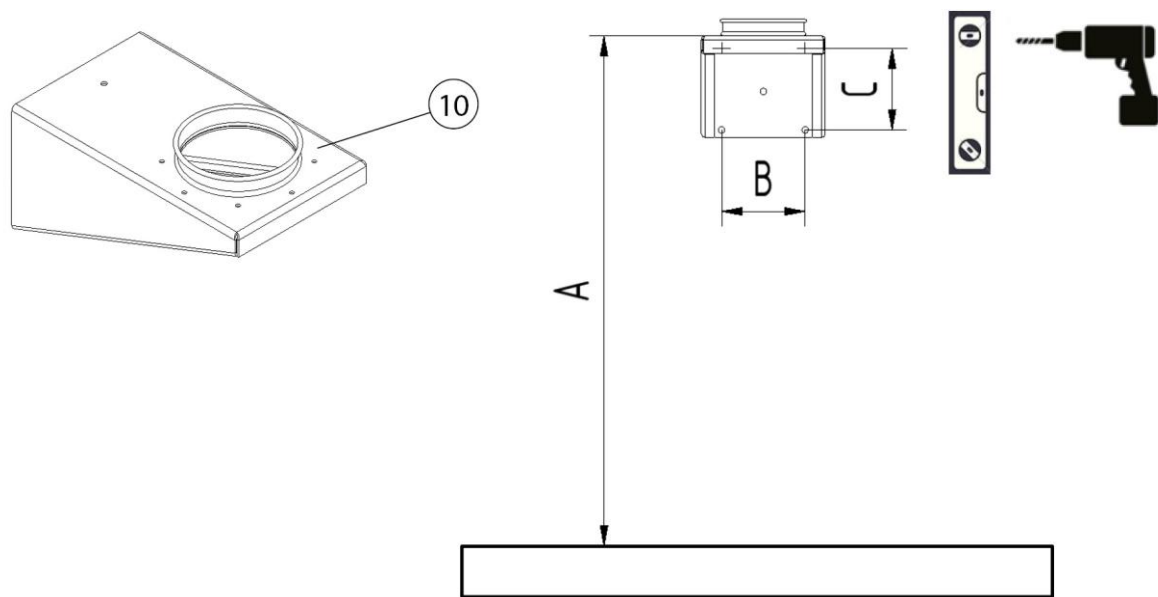
Abb. 4: Bohrbild
